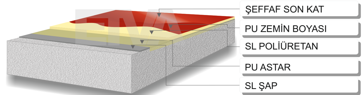
Kaplama kalınlığı ~ 2,5 mm
